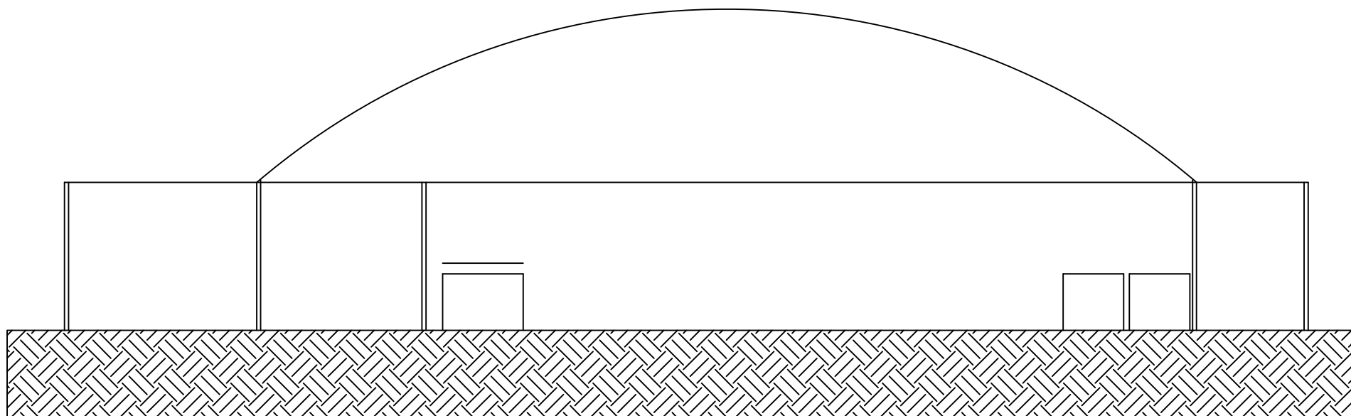
Fachada Esc.:1/200
