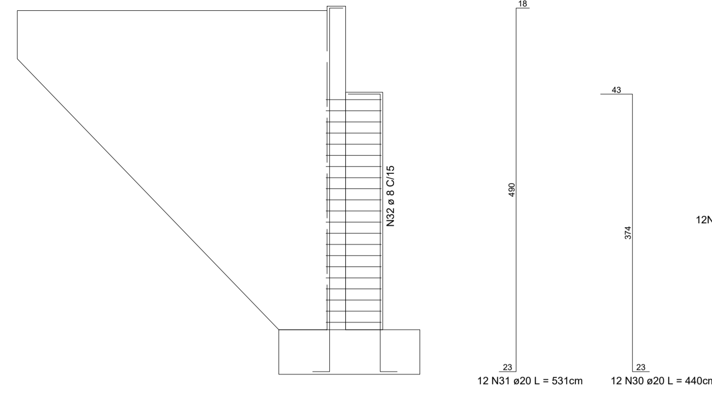
PILARES - ARMADURAS - CORTE BB
