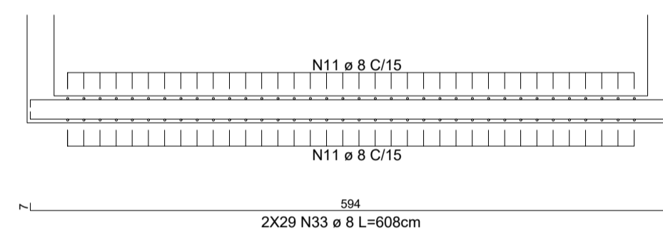
CORTINA - ARMADURAS - CORTE EE
