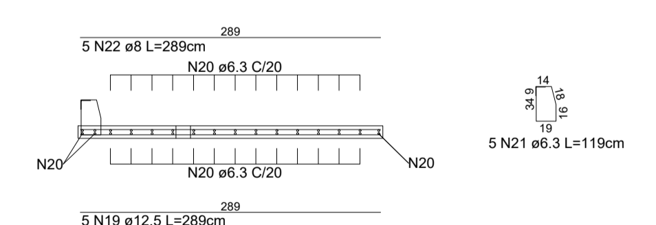
LAJOTA PRÉ-MOLDADA ELEVÇÃO
