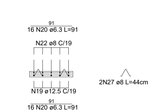
LAJOTA PRÉ-MOLDADA CORTE FF
