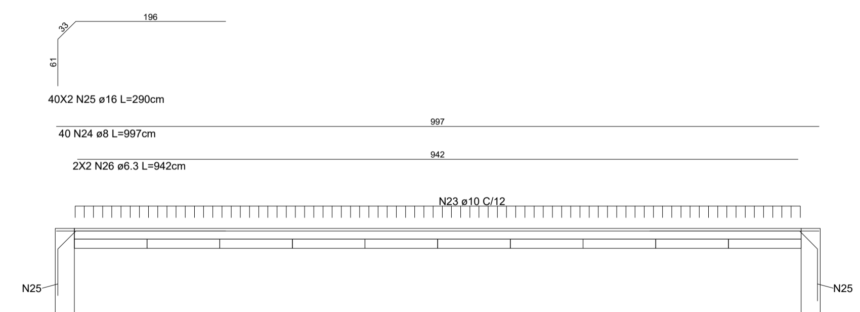
LAJE - ARMADURAS - CORTE LONGITUDINAL
