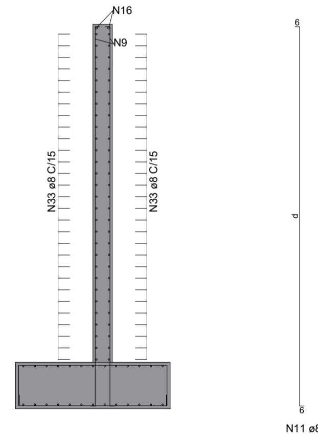
CORTINA - ARMADURAS - CORTE DD
