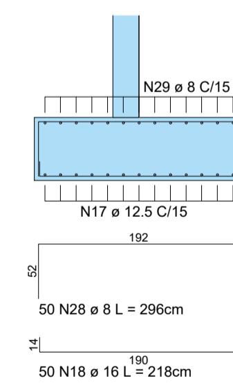
SAPATA - ARMADURAS - CORTE GG
