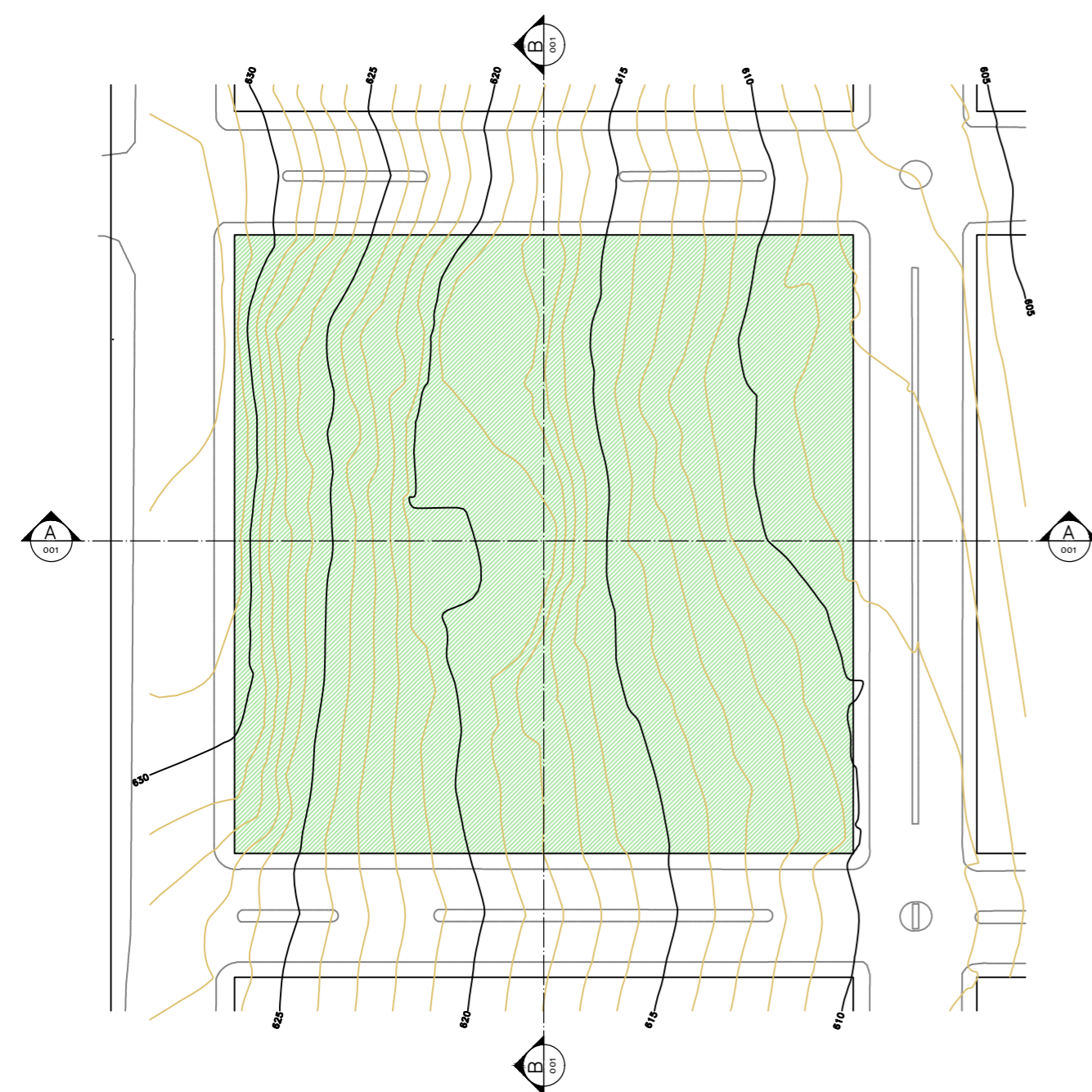
ALTIMETRIA Esc.: 1 : 1000
