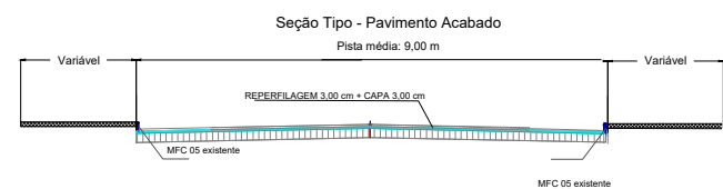
Seção Tipo - Pavimento Acabado - Rua Edson Giacomelli
