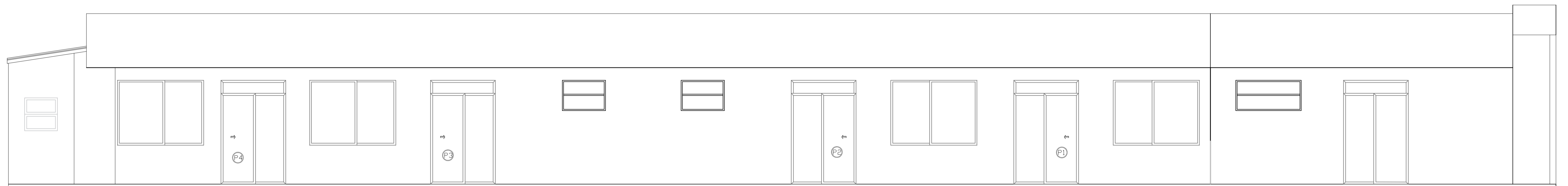
FACHADA 3 ESC.: 1:75
