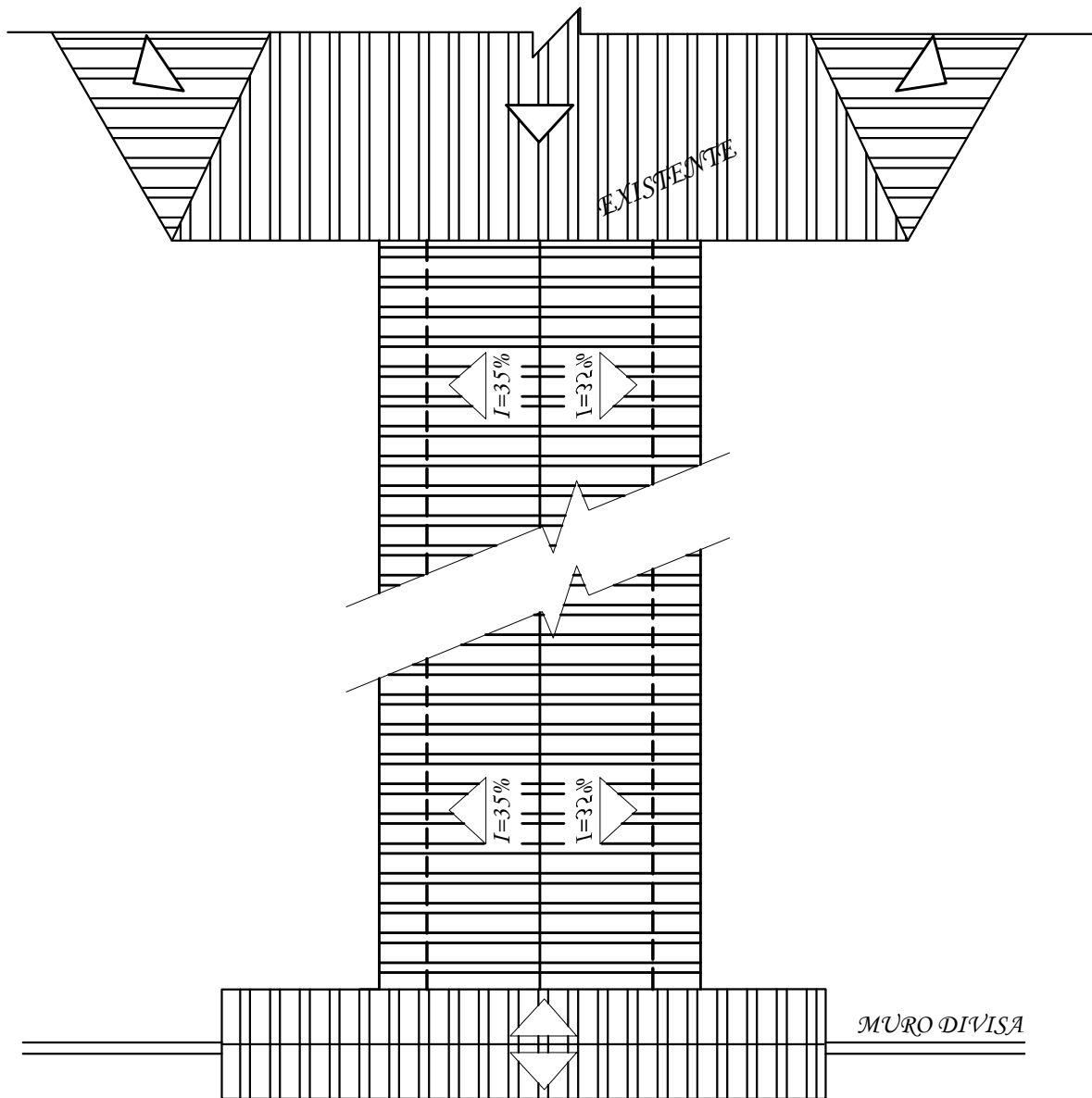
PLANTA DE COBERTURA ESC.: 1:150
