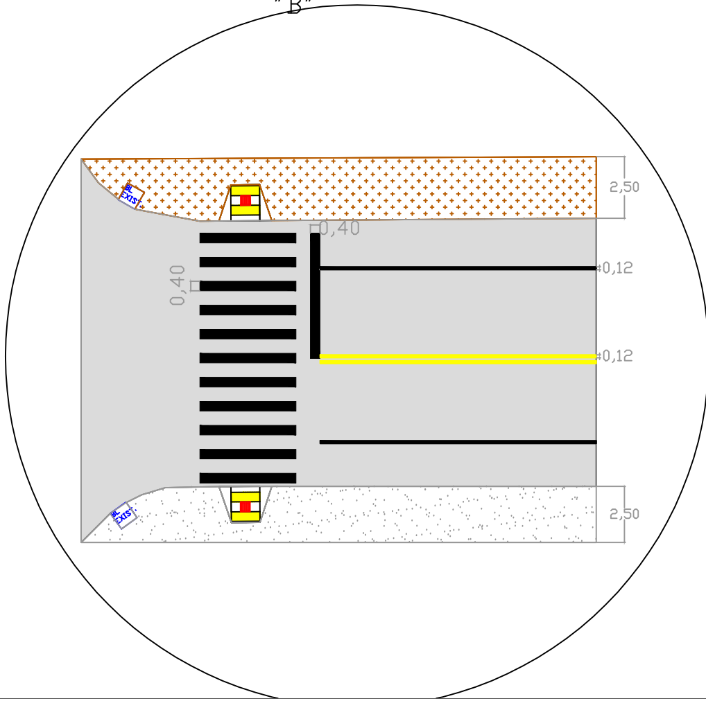
DETALHE "B"
